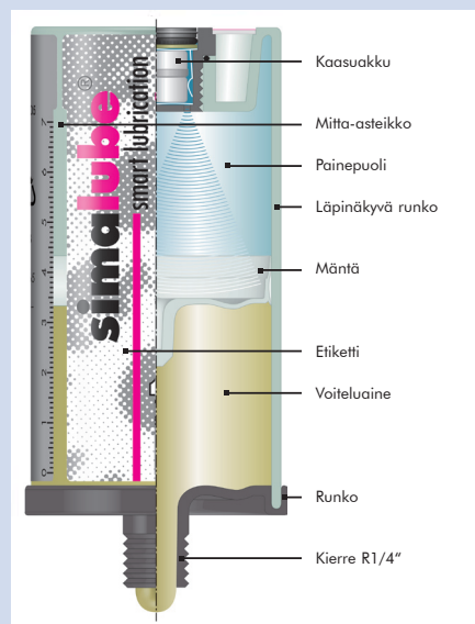
Hytin rasvanippa jonka tilalle voidaan asentaa simalube® voiteluannostelija
