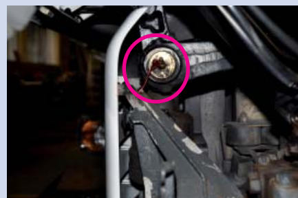
Hytin rasvanippa jonka tilalle voidaan asentaa simalube® voiteluannostelija
